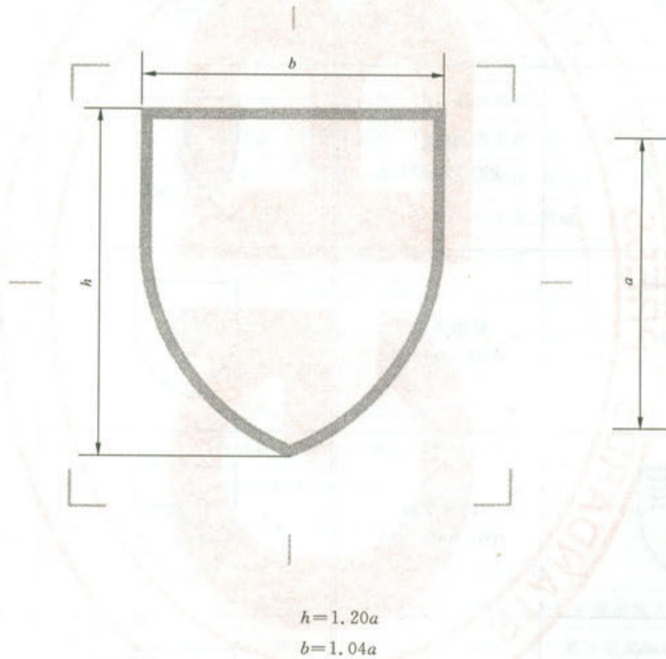
图 B.1 ISO 7000-2410 防护的基本图形符号
